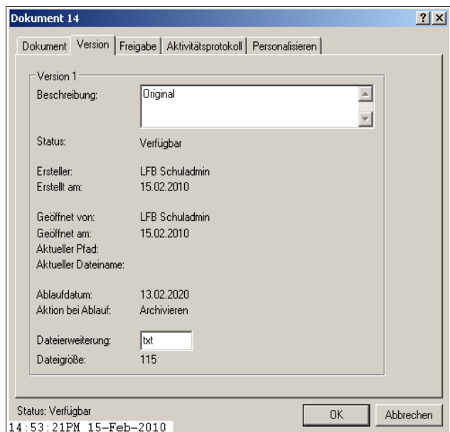
Abbildung 11: Versionsnummer
