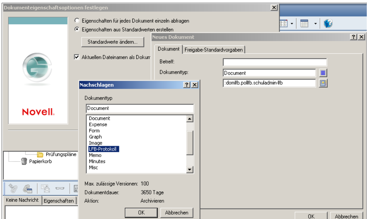
Abbildung 5: Dokumenttyp anpassen
