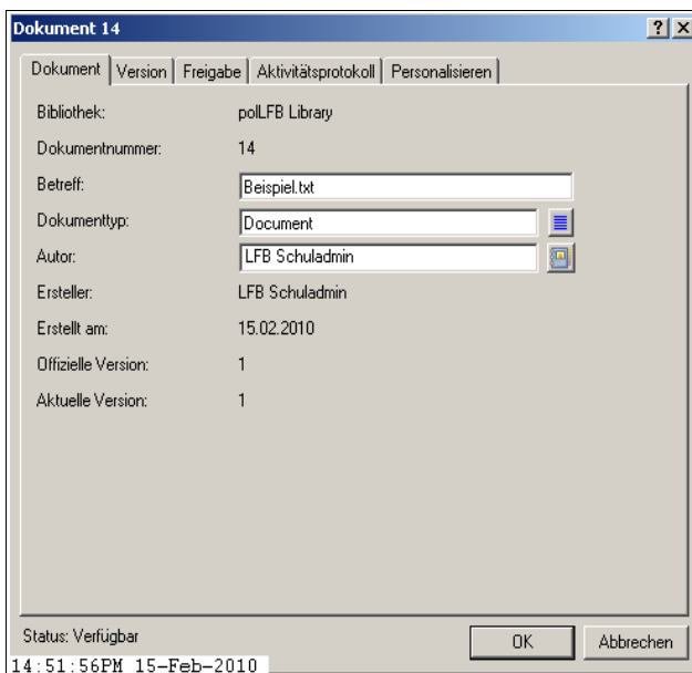
Abbildung 10: Dokumenteigenschaften
