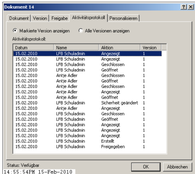
Abbildung 13: Aktivitätsprotokoll
