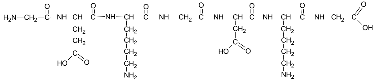
Molekülstruktur Gelatine (beispielhafte Kette)
