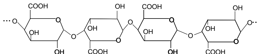
Kette aus \alpha -D-Galacturonsäure-Bausteinen
