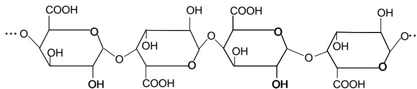
Molekülstruktur Pektin (beispielhafter Kettenausschnitt)
