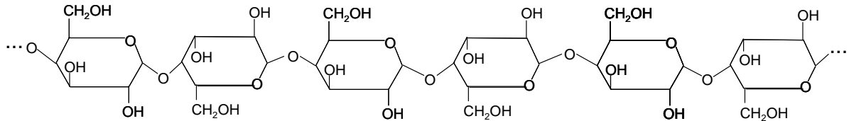
Molekülstruktur Agar-Agar (vereinfachter Kettenausschnitt)
