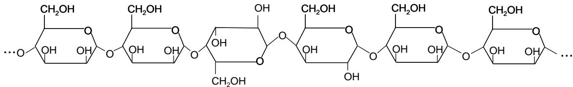
Molekülstruktur Johannisbrotkernmehl (beispielhafter Kettenausschnitt)
